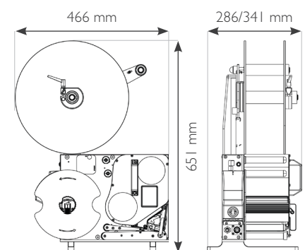
Abmessungen
